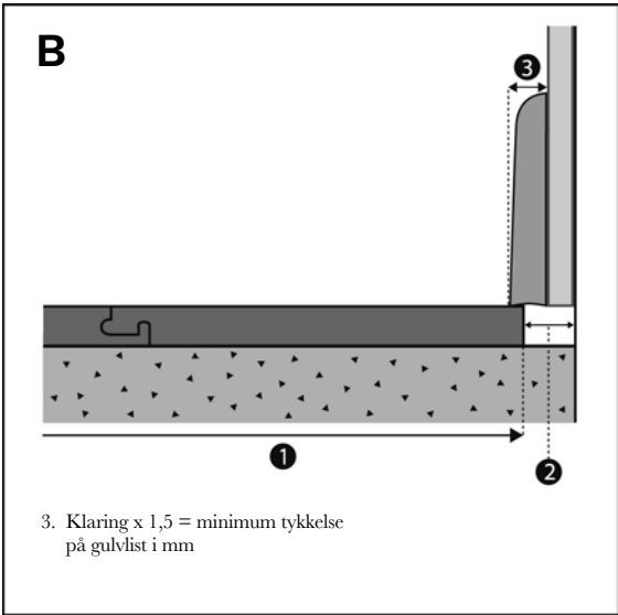
Påse at gulvet kan bevege seg fritt under veggplatene.
